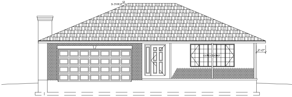
FRONT ELEVATION A-1 SCALE: 1/4"=1'-0"
